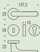
CC11 R-RY Ø50
