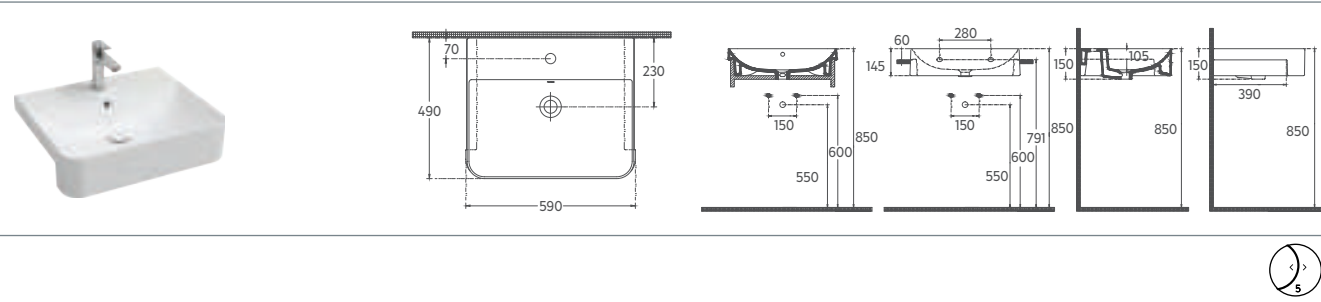
SOTT’AQUA Yarım Countertop Washbasin, 59 cm
