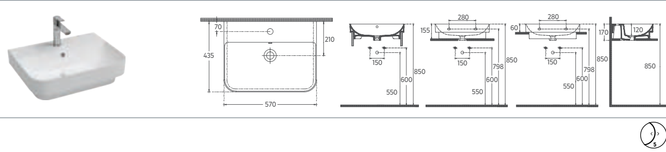
SOTT’AQUA Inset Washbasin, 57 cm
