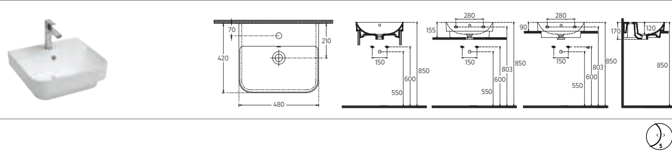
SOTT’AQUA Inset Washbasin, 48 cm
